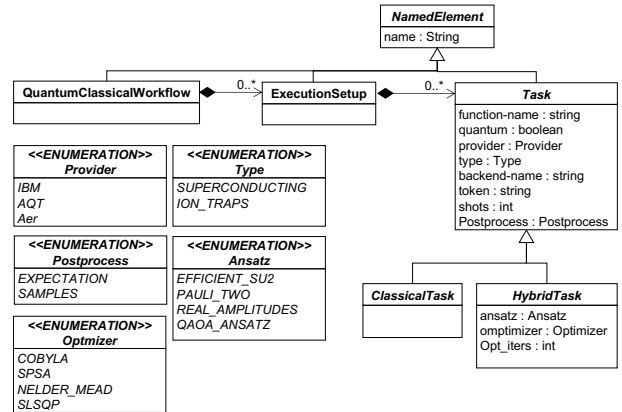
Fig. 4: RIGOLETTO metamodel.
